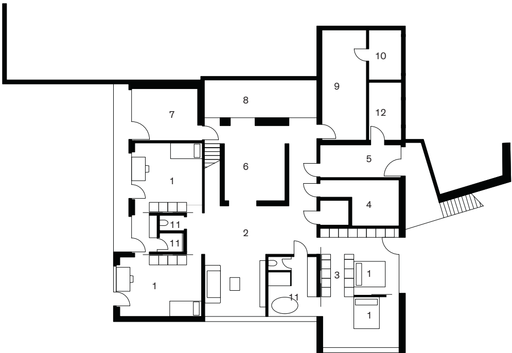
Grundriss EG
